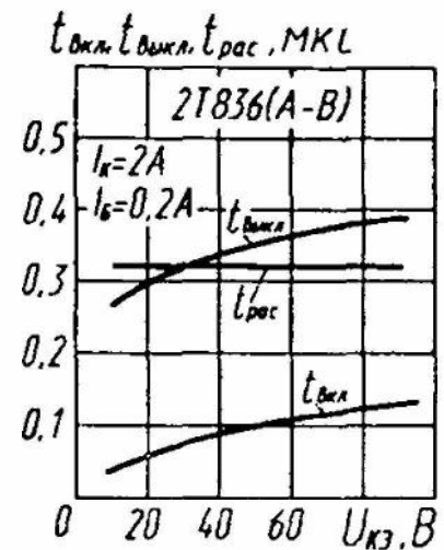
Зависимости времени включения, выключения, и рассасывания от напряжения коллектор—эмиттер
