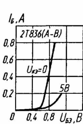
Входные характеристики
