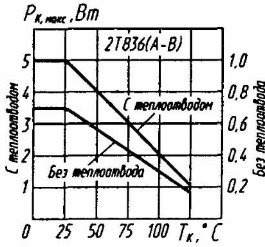
Зависимость максимально допустимой постоянной рассеиваемой мощности коллектора от температуры корпуса
