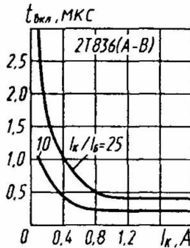
Зависимости времени включения от тока коллектора
