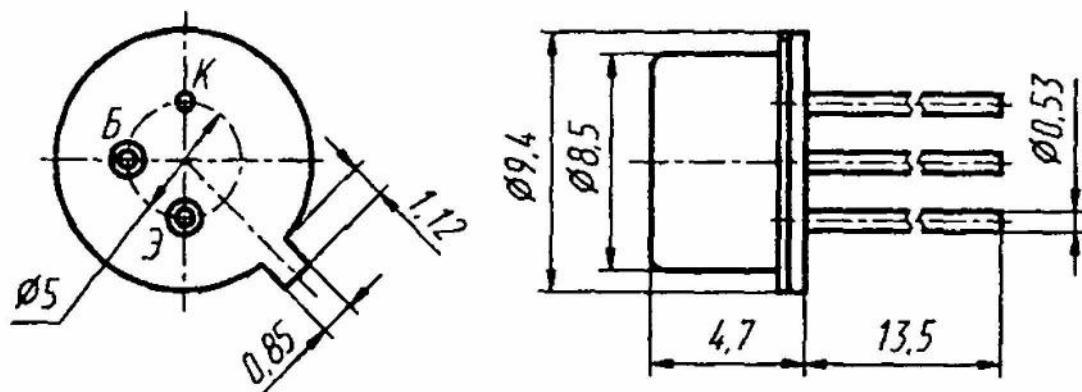
2Т836А-5
