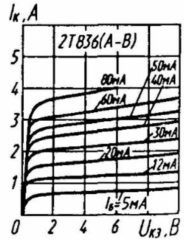
Выходные характеристики
