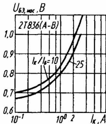
Зависимости напряжения насыщения база-эмиттер от тока коллектора
