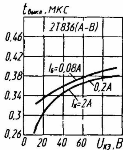
Зависимости времени выключения от напряжения коллектор-эмиттер
