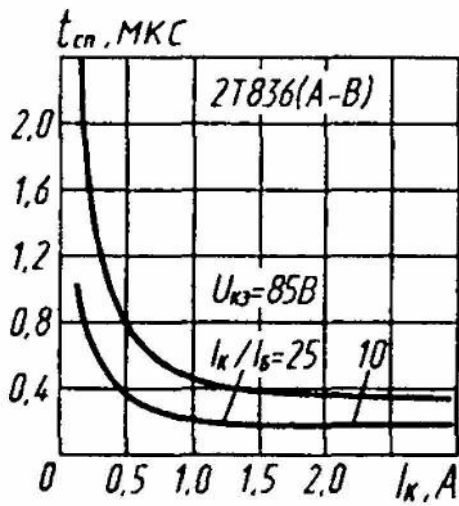
Зависимости времени спада от тока коллектора
