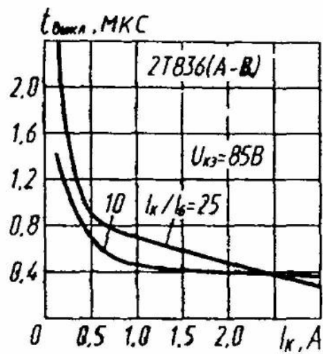
Зависимость времени выключения от тока коллектора
