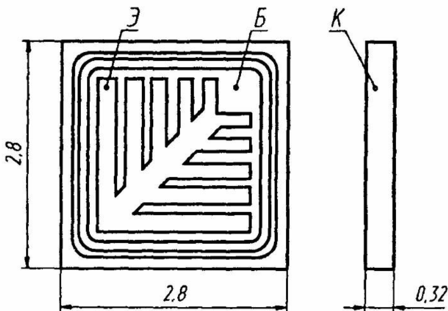
2Т836А-5
