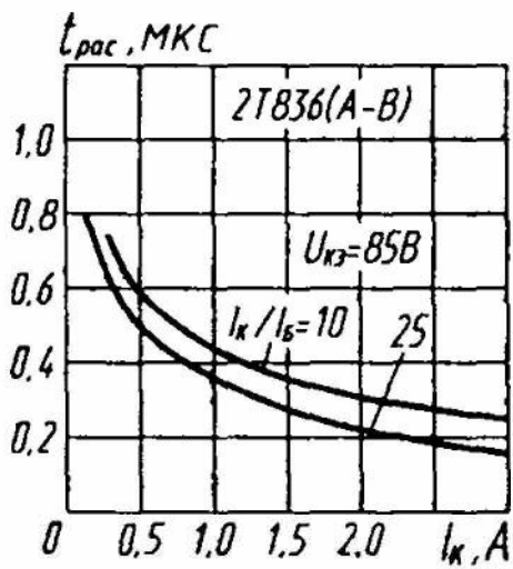
Зависимости времени рассасывания от тока коллектора
