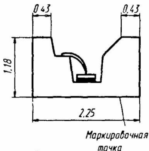
2Т3115А-6
