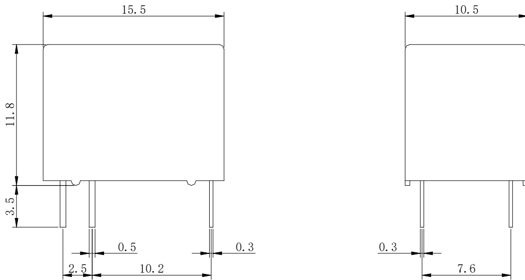
PC Board layout 安装图
