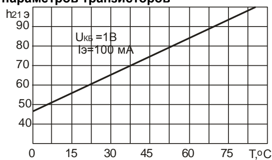
Зависимость статического коэффициента передачи тока от температуры
